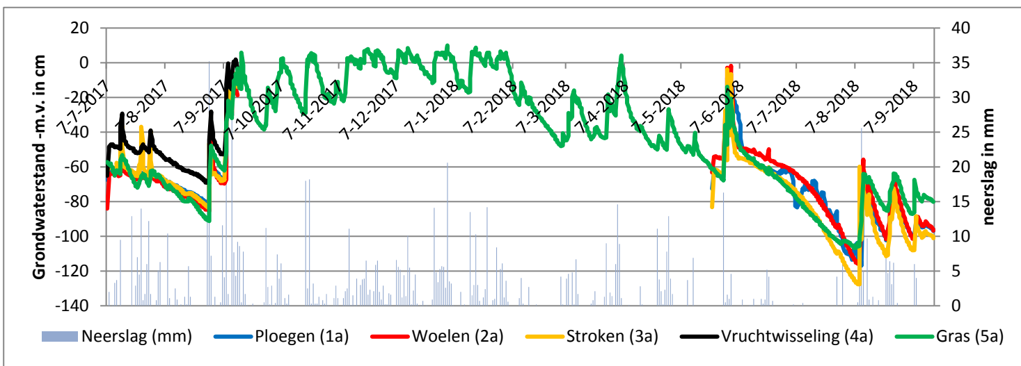
Figuur 9. Verloop van grondwaterstanden in 2017 en 2018 op het voorstel deel van het perceel (herhaling 1). In de winter van 2017-2018 is enkel de grondwaterstand onder het grasobject gemeten.
