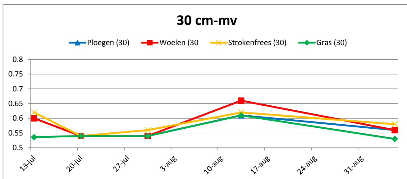
Figuur 17. Vochtgehalten in de bodem in de verschillende systemen op 30 centimeter onder maaiveld.
