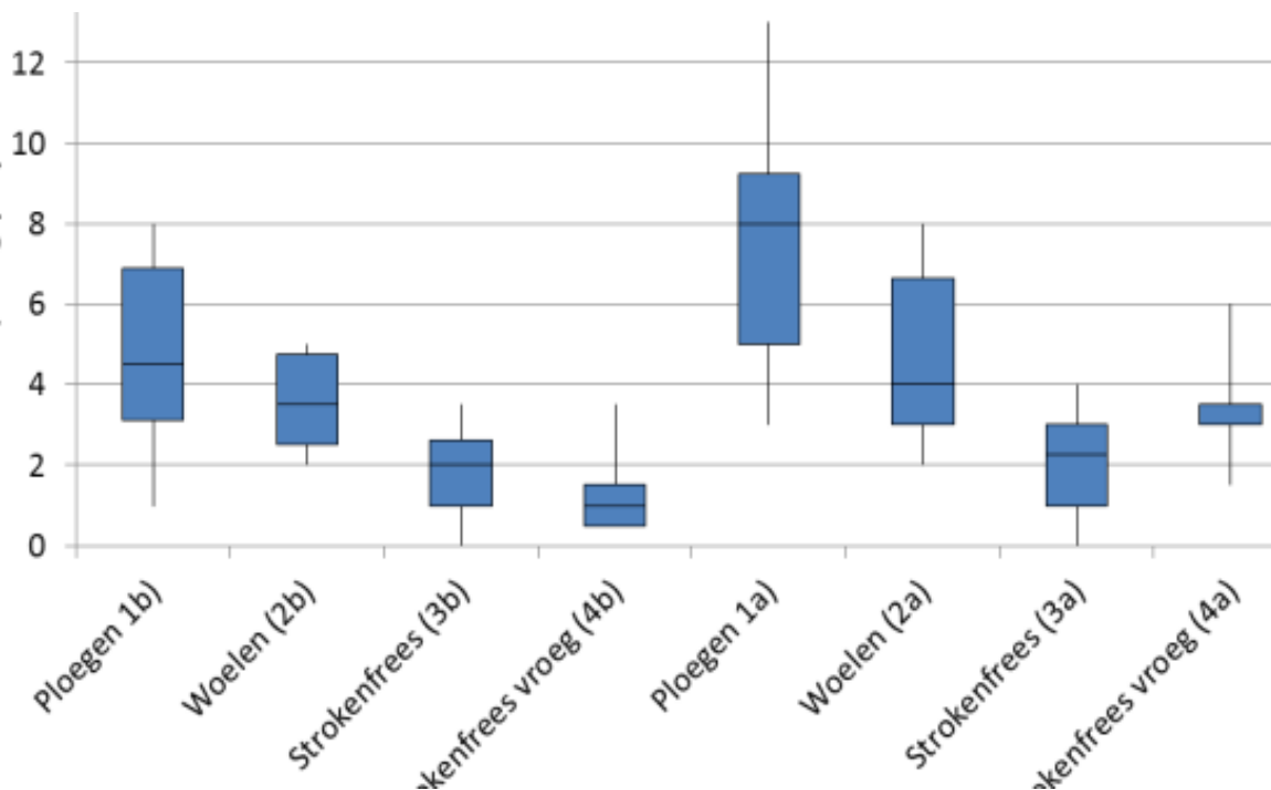
Figuur 13. Gemeten insporing in de verschillende objecten. De letters a en b geven de herhalingen aan.
